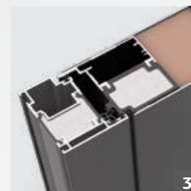
Dodatna izolacija v konstrukciji
